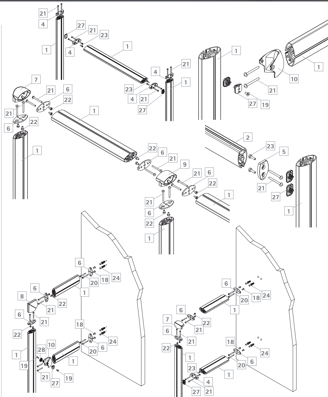
IT dado ad incastro, per montare pannelli leggeri con viti autofilettanti DE einklickmutter, für montage leichter paneele mit blechschrauben EN nut, to mount lightweight panels with self tapping screws
